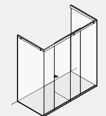
Flat D – F2 Esempio di doccia a tre lati con anta scorrevole example for shower with three sides and sliding door
