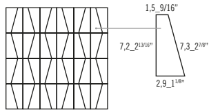
SIDE_29,6X29,6 11 5/8" x 11 5/8"
