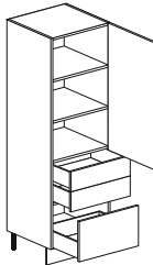
p 600 - 1 anta, 2 cassetti, 1 estrattore, ripiani l 450, 600 d 23 5/8" - 1 door, 2 drawers, 1 puller, shelves w 17 11/16", 23 5/8"
