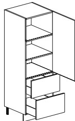
p 600 - 1 anta, 2 estrattori, ripiani l 450, 600 d 23 5/8" - 1 door, 2 pullers, shelves w 17 11/16", 23 5/8"
