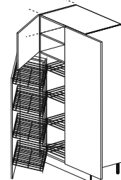
p 600 - angolo, 1 anta, 1 struttura estraibile, 1 ripiano l 1250, 1287, 1350 d 23 5/8" - corner, 1 door, 1 pull-out structure, 1 shelf w 49 3/16", 50 11/16", 53 1/8"
