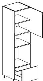
anta, 1 estraattore, ripiani, vano forno l 600 door, 1 puller, shelves, oven unit w 23 5/8"
