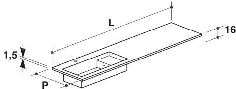
Piani con lavabo integrato Top with built-in basin
