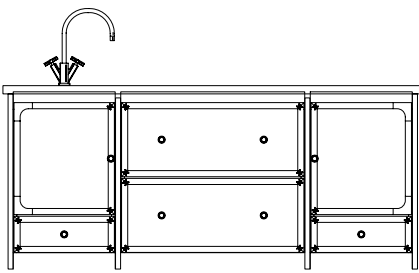
1908 ISLAND UNIT W. 204cm, D. 140cm, H. 90cm
