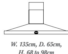
W. 135cm, D. 65cm, H. 68 to 98cm
