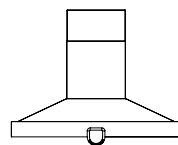
CORNUFE 110 W. 110cm, D. 65cm, H. 70 à 98cm Extraction rate: 1000m³/h
