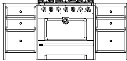
1908 ISLAND UNIT W. 204cm, D. 110cm, H. 90cm
