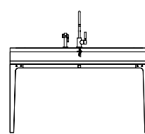
SINK W. 150cm, D. 70cm, H. 75cm Piètement seul
