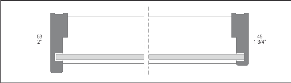
SEZIONE ANTA - DOOR SECTION
