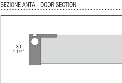
complanare - coplanar door
