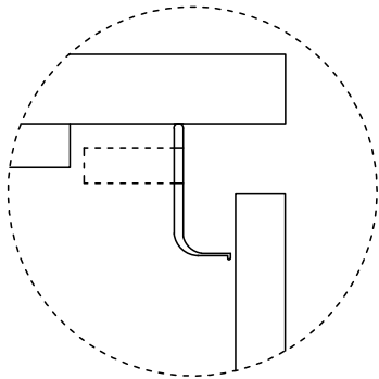
GOLA L
