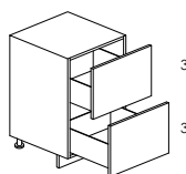
BAJO 2 GAVETAS 40/45/50/60/70/80/90 /100/120
