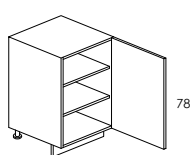
BAJO 1 PUERTA 15/20/25/30/35/40/45 /50/60
