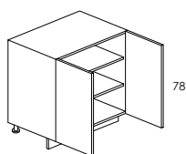
BAJO 2 PUERTAS 70/80/90/100
